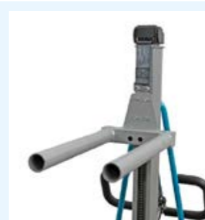
Rollengabel für die Modelle E-MES100-17/150-15 und MES100-15/200-15
